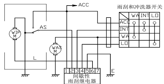
电路图
